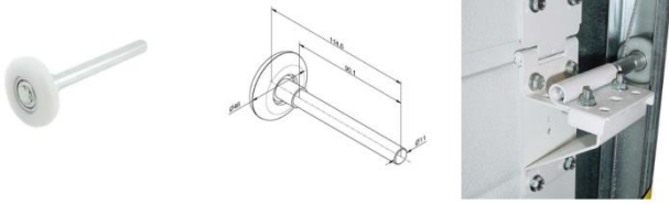
Rolă
