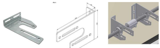
Suport arc
