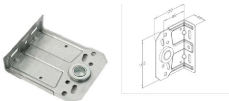
Suport ax
